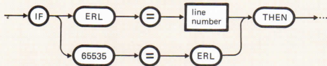
Figure 13-8 ERL Function
